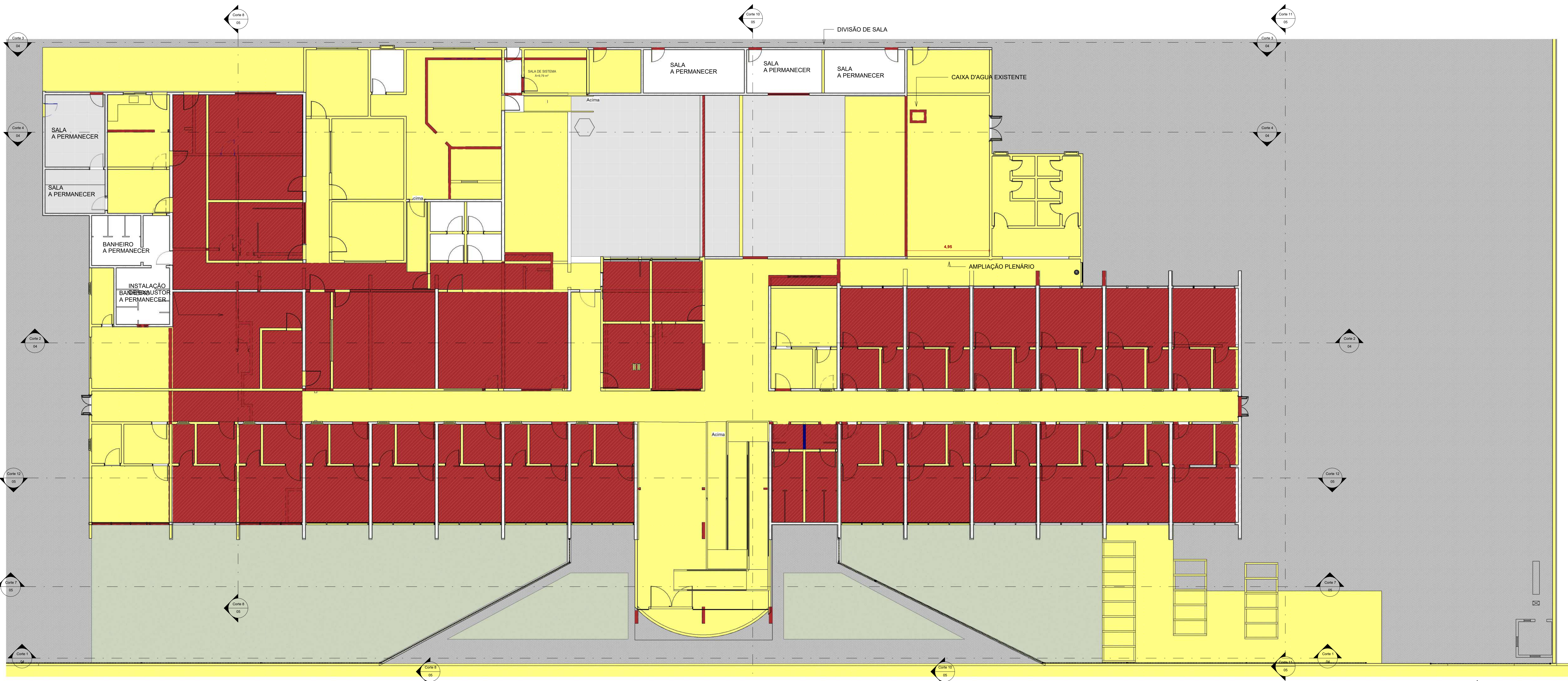
1 Planta de construir / demolir Escala: 1 : 100
